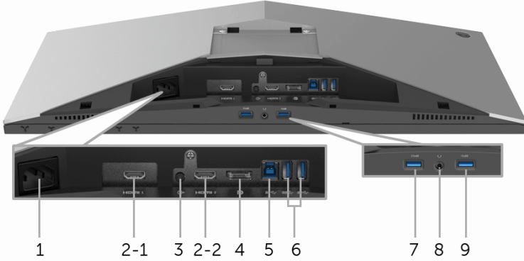
المنظر الخلفي والأمامي بدون حامل الشاشة
